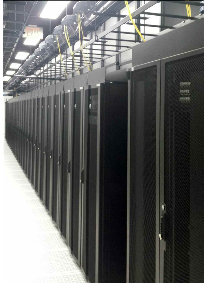
配置垂直排风管的 CPI GF 系列 GlobalFrame 机柜是 Cologix 整体解决方案（温哥华站点）的一部分。
