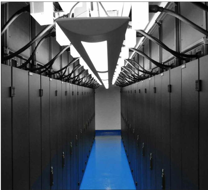
CPI 的被动型数据中心散热解决方案可隔离热空气，同时容纳架空电力总线槽。
