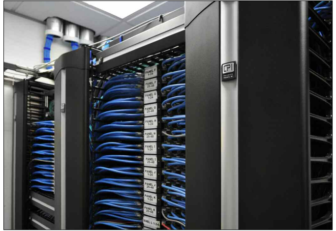
Evolution 缆线管理用于所有 Scripps 的 IDF 设备间，以在移动、添加和更改时节省时间和金钱。
